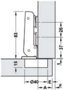
Schiță de găurire
