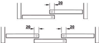
Dimensiuni suprapunere uși
