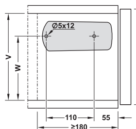
Montaj orizontal
