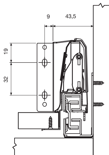
Cote montaj suport spate
