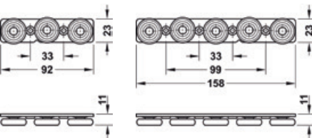
Role sistem culisare liniară 29 mm
