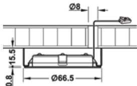
Montaj aplicat
