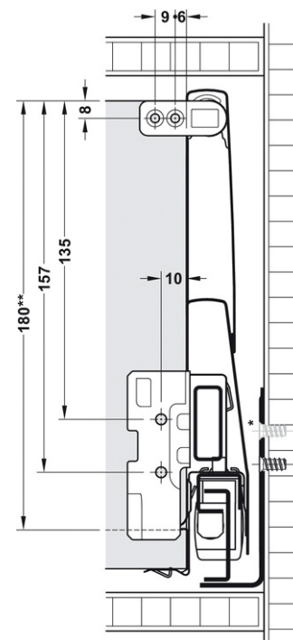
Cote standard prelucrare spate, lătală 115 mm
