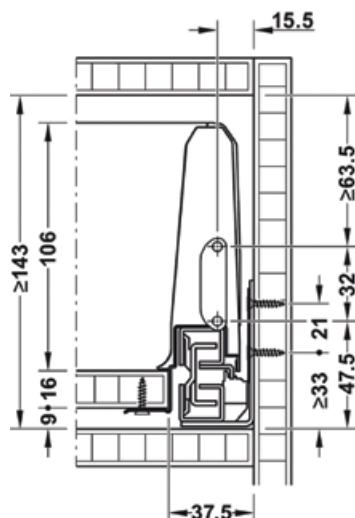
Cote montaj cuplaj front
