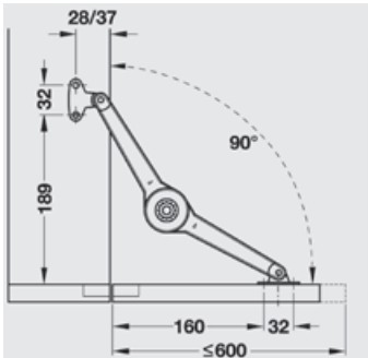
Duo Forte coborâre, montare ușă bar - Tabel referință unghi de deschidere 90°
