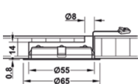
Montaj încastrat
