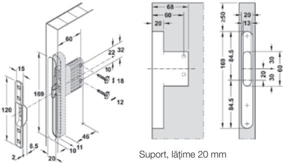
Suport, lățime 20 mm
