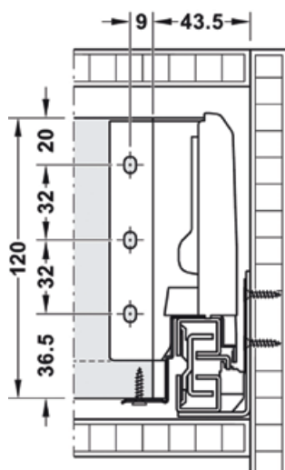
Cote montaj suport spate
