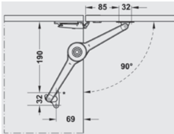
Duo Forte Push front fără mâner, montare pentru susținere ușă - Tabel referință unghi de deschidere 90°
