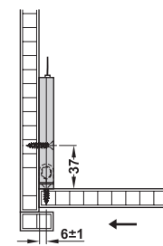
Ușă culisantă încadrată
