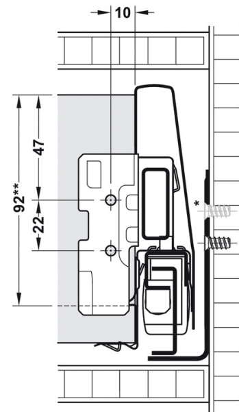
Cote prelucrare spate laterală 115 mm
