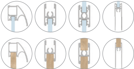
Posibilitate combinare materiale în profiluri
