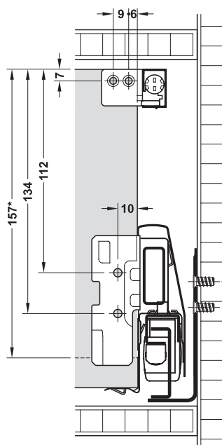
Cote standard prelucrare spate, laterală 92 mm
