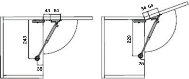
Cote de montaj pentru aplicații la 90° și 110°
