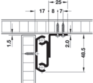
Sarcină 90 kg
