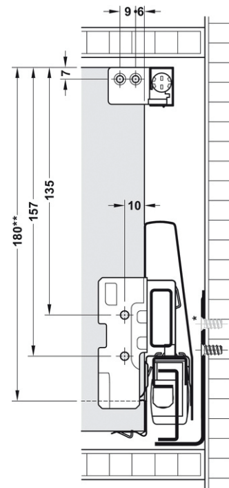
Cote standard prelucrare spate, laterală 115 mm
