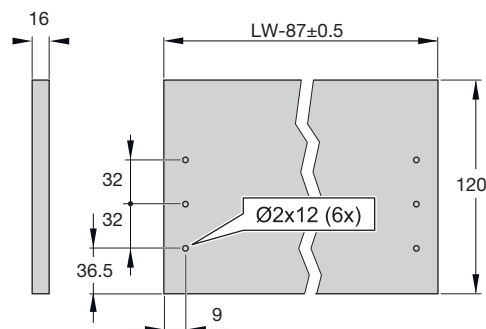
Cote prelucrare spate
