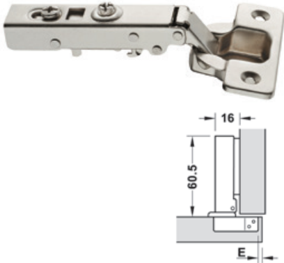
Cote găurire cupă balama ușă aplicată
