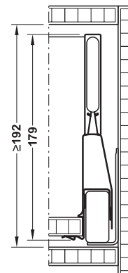
Laterală 92 mm + element inserție laterală
