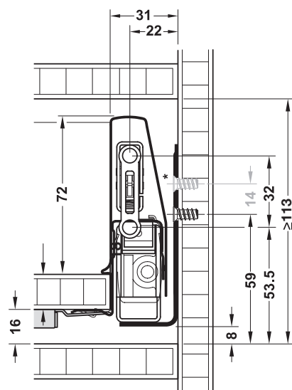
Cote prelucrare front
