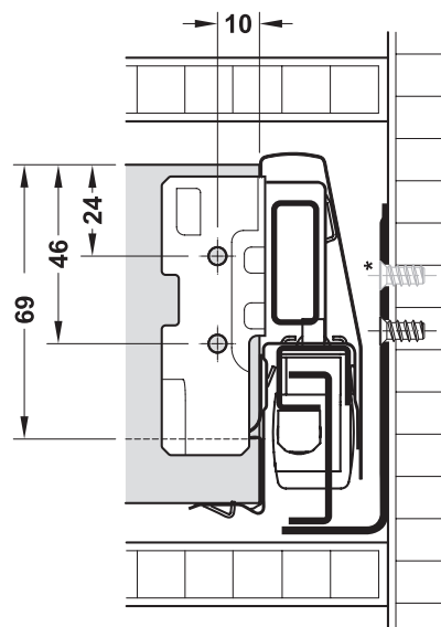
Cote prelucrare spate laterală 92 mm
