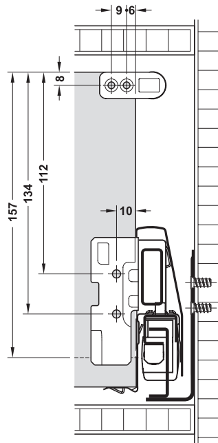
Cote standard prelucrare spate, laterală 92 mm
