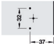
Schiță de găurire
