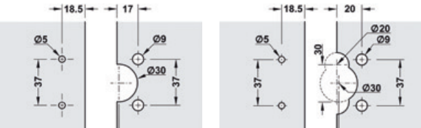
Acoperire 3 mm
