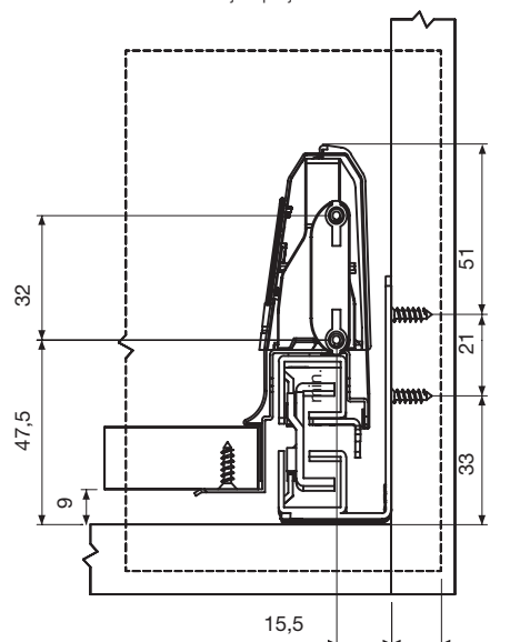
Cote montaj cuplaj front
