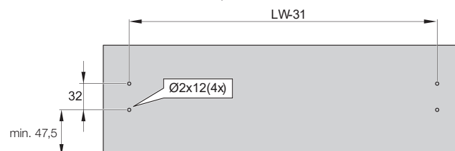
Cote prelucrare front
