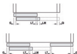
Dimensiuni suprapunere uși
