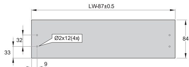
Cote prelucrare front
