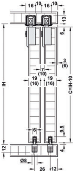
Dimensiuni montaj în canal Pentru montaj prin lipire
