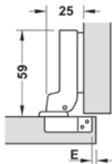
Cote găurire cupă balama ușă semiaplicată
