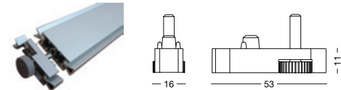
Picior profil, reglabil
