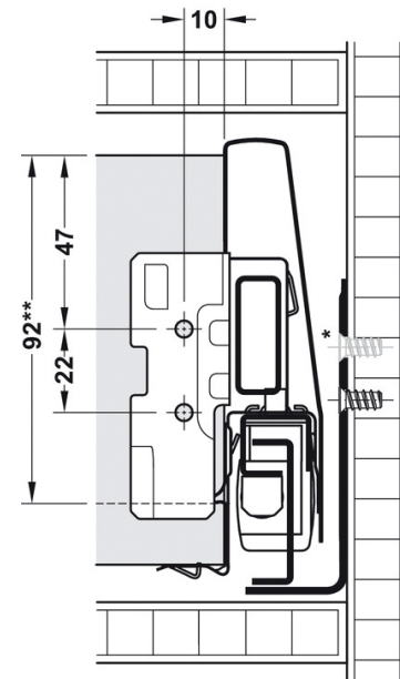
Cote prelucrare spate laterală 115 mm
