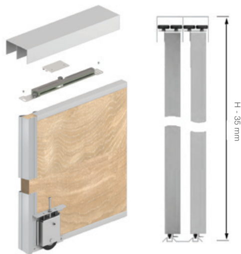
Detaliu componente sistem U-18 STANDARD
