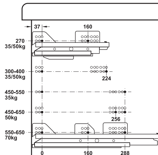
Schiță de găurire
