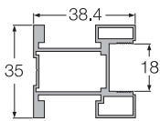
Secțiune profil mâner
