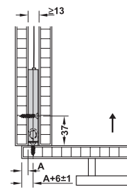
Sertar cu încuietoarea montată în lateral
