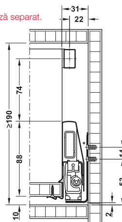
Cote prelucrare front
