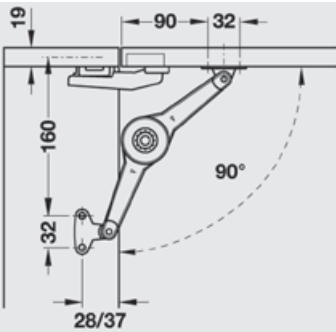
Duo Standard front cu mâner, montare pentru susținere ușă - Tabel referință unghi de deschidere 90°
