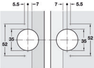
Schiță de găurire
