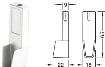
Suport pentru capăt închis
