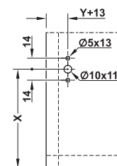
Reglarea mecanismului
