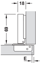
Balama Metalla 300 SM Mini 95° CLIP ușă semiaplicată
