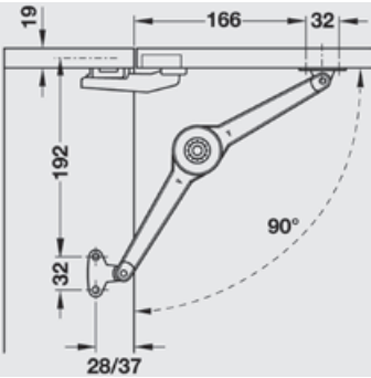
Duo Forte front cu mâner, montare pentru susținere ușă - Tabel referință unghi de deschidere 90°
