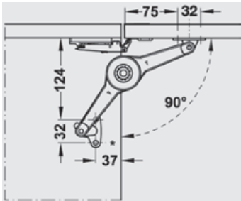
Duo Standard Push front fără mâner, montare pentru susținere ușă - Tabel referință unghi de deschidere 90°
