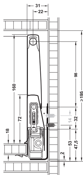
Cote standard prelucrare front, lătală 92 mm
