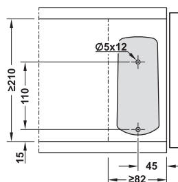
Montaj vertical
