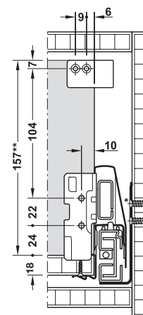
Cote prelucrare spate
