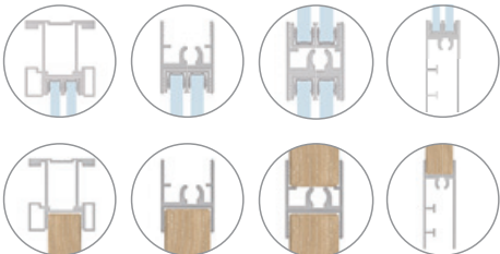
Posibilitate combinare materiale în profiluri
