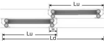
Calcul suprapunere uși
