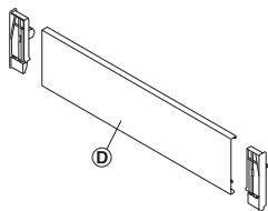
Lungime front (D) = lățime interioară corp - 10 mm
