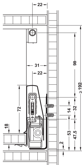
Cote standard prelucrare front, laterală 92 mm
