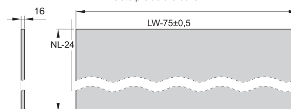
Cote prelucrare bază
