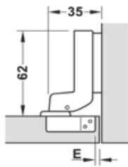
Cote găurire cupă balama ușă încadrată
