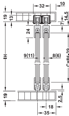
Cu profil fixare sticla la partea inferioară Pentru montaj prin lipire
