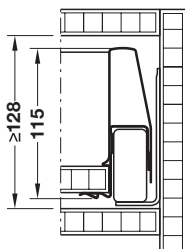
Laterală 115 mm
