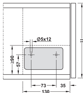
Montaj orizontal
