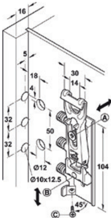
Suport scurt
