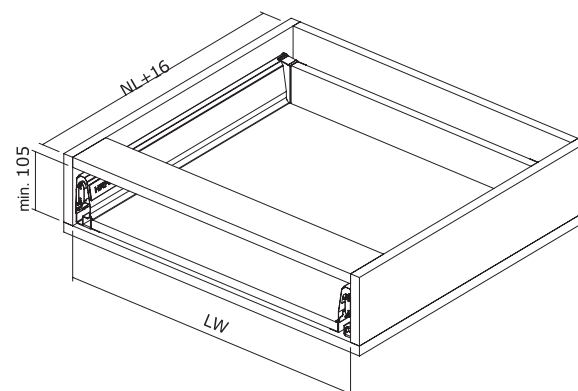
Spațiu necesar instalare
