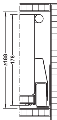
Laterală 92 mm + lonjeron dreptunghiular sau rotund
