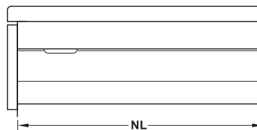
Adâncime minimă instalare = NL + 3 mm NL = Lungime nominală glisieră / laterale
