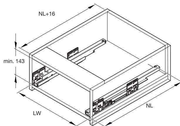
Spațiu necesar instalare
