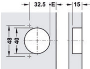
Schiță de găurire
