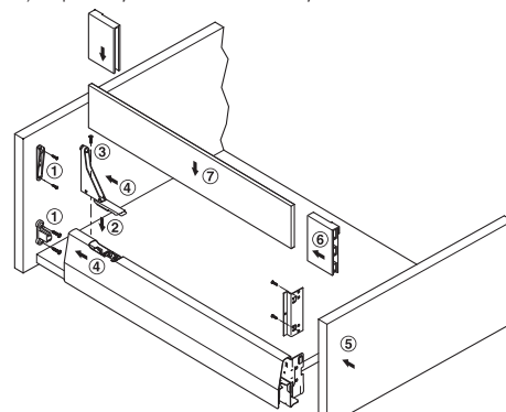
Montaj element inserție
