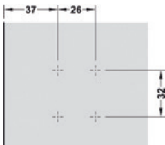
Schiță de găurire
