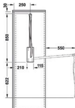
Instalare pe rândul de găuri central
