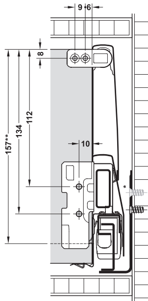
Cote standard prelucrare spate, lătală 92 mm
