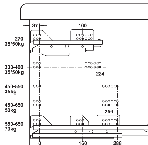
Schiță de găurire
