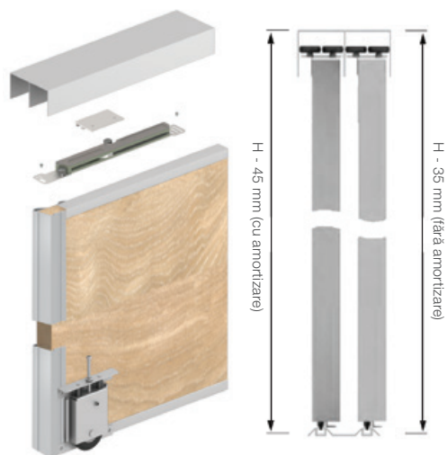
Detaliu componente sistem Eco
