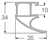
Secțiune profil mâner
