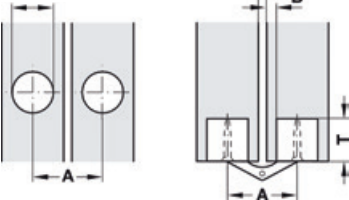
Schiță de găurire
