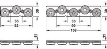
Role sistem culisare liniară 39 mm
