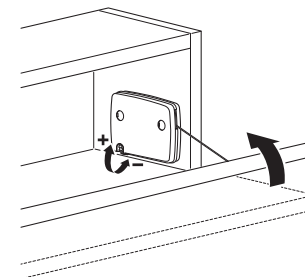
Reglarea mecanismului
