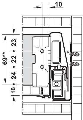
Cote prelucrare spate
