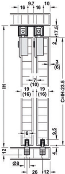
Dimensiuni montaj prin înșurubare
