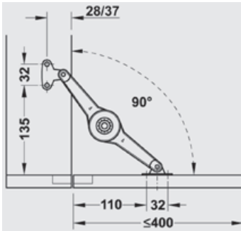
Duo Standard coborâre, montare ușă bar - Tabel referință unghi de deschidere 90°
