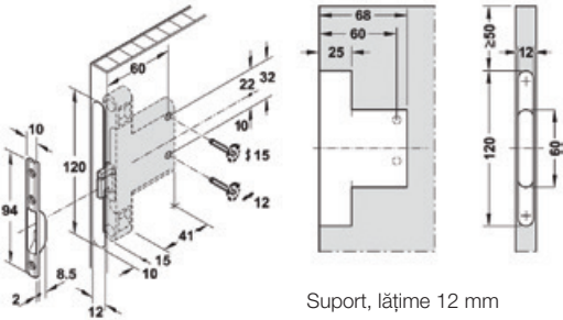
Suport, lățime 12 mm
