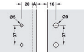
Schiță de găurire
