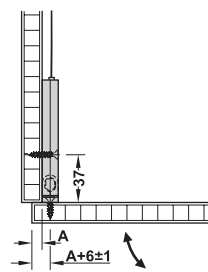
Ușă cu balamale aplicate
