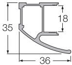
Secțiune profil mâner
