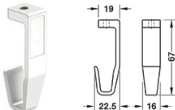
Suport central
