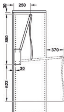
Instalare pe rândul de găuri din spate
